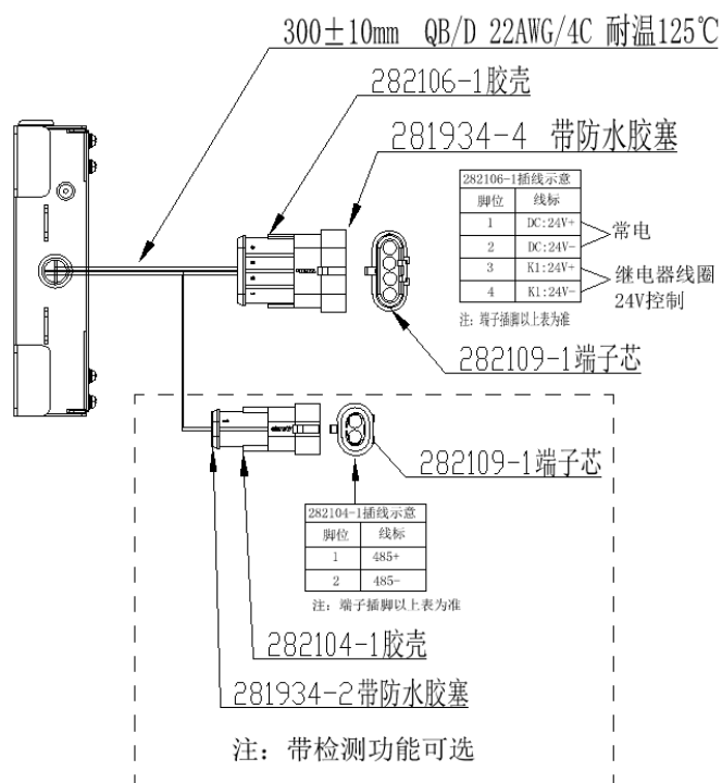
图 2 带检测功能接线示意图
