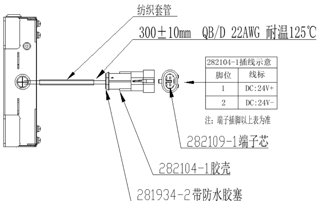
图 3 不带检测功能接线示意图
