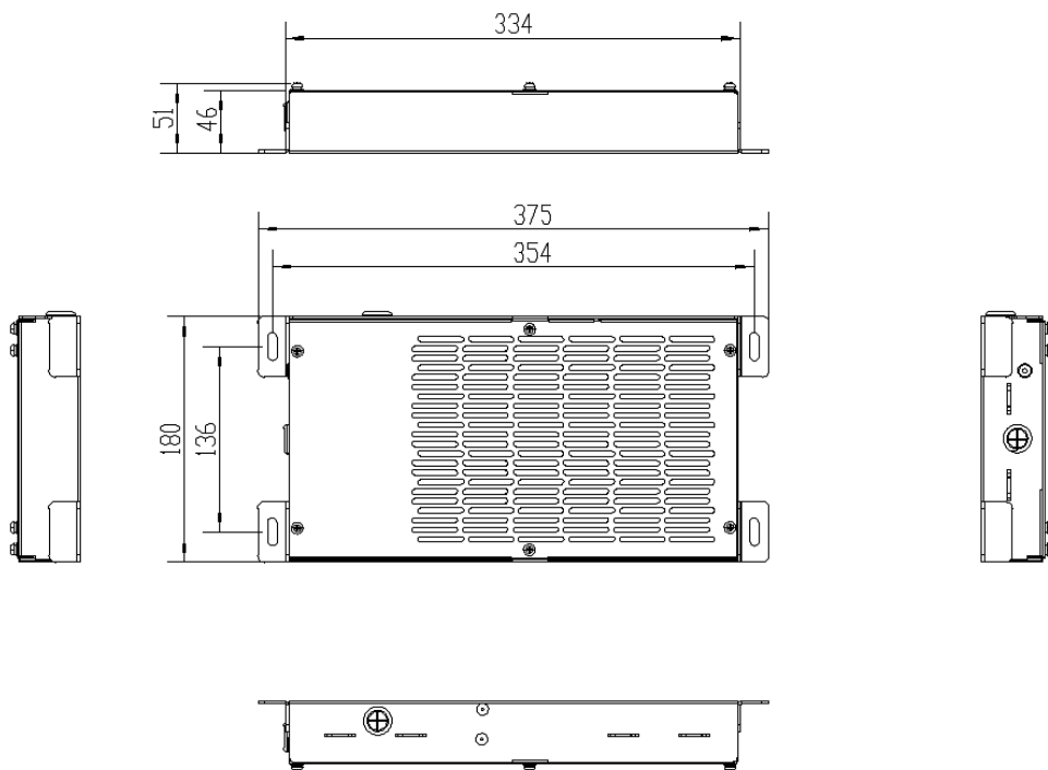
图 1 外形图
