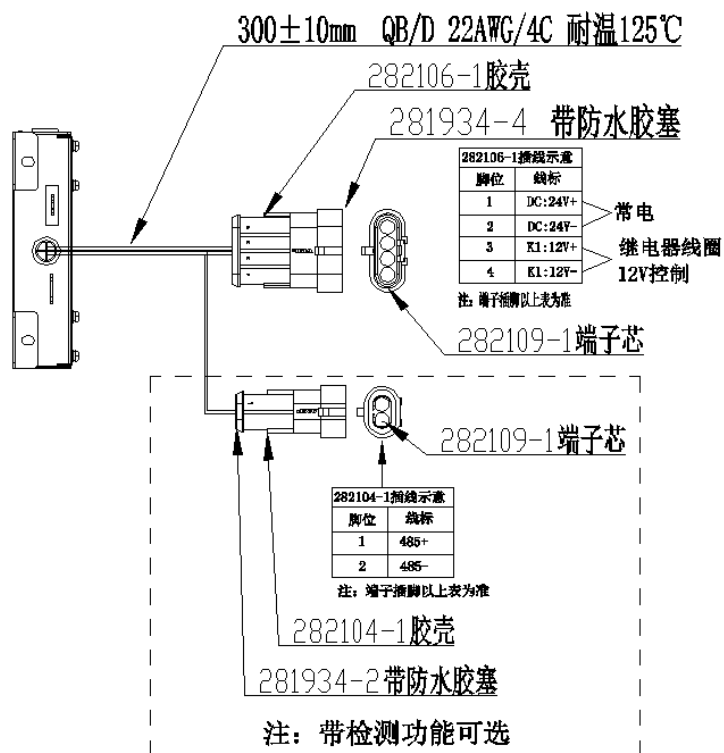
图 4 控制开关 12V
