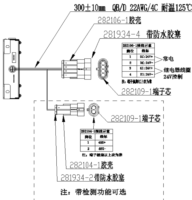
图 3 控制开关 24V
