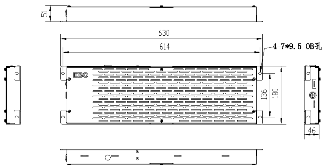
图 1 外形尺寸图 (不带工作指示灯)
