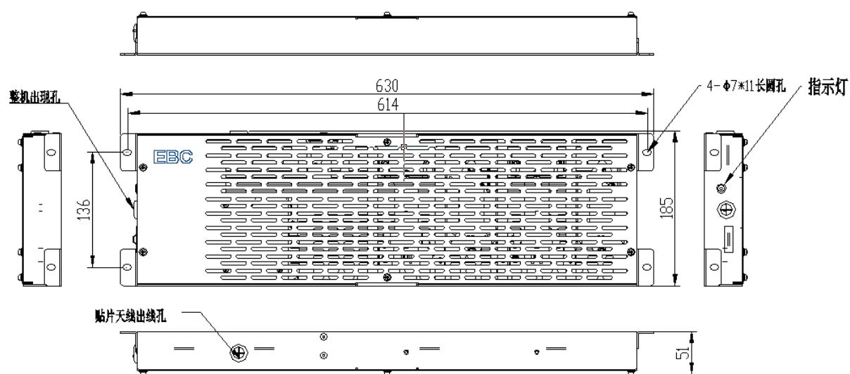
图 2 外形尺寸图 (带工作指示灯)
