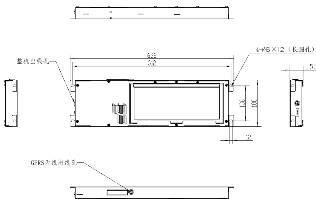
图 1 外形尺寸图 (632*180*51mm)
