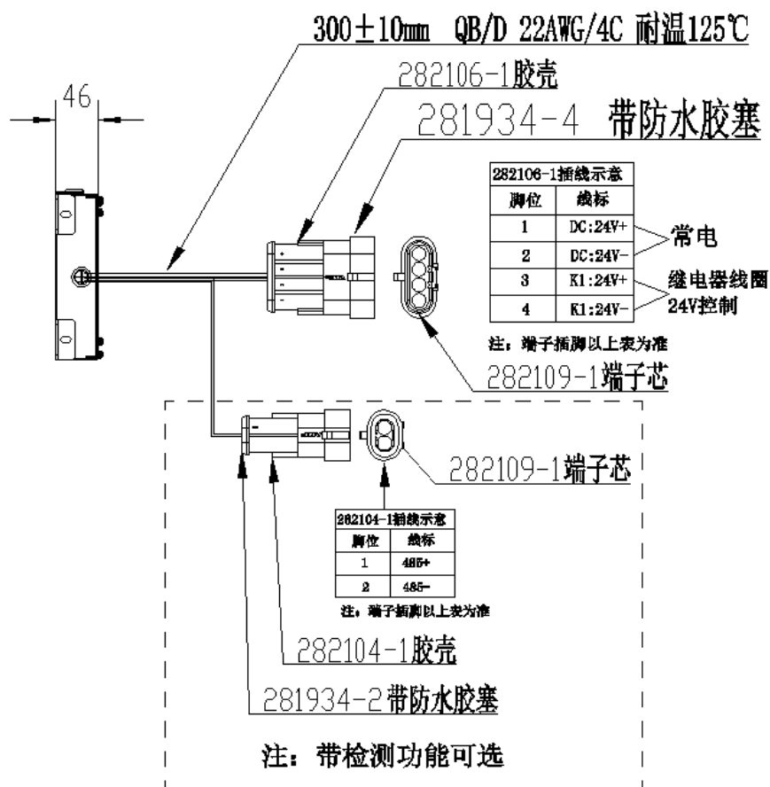
图 5 对接 4P 端子接线示意图 (可选带 485 通)
