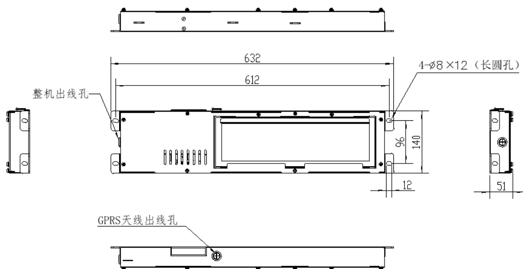
图 2 外形尺寸图 (632*140*51mm)
