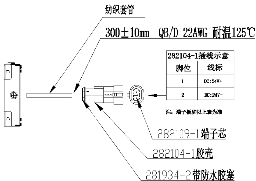
图 3 对接 2P 端子接线示意图
