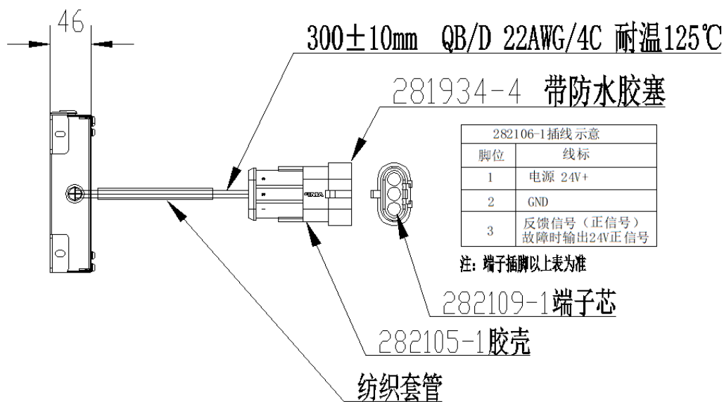
图 4 对接 3P 端子接线示意图
