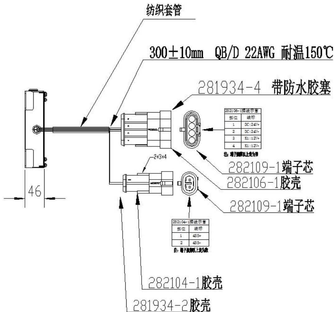
图2 12V 控制电源连接空调示意图
